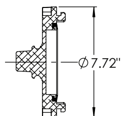
Storz Cap
